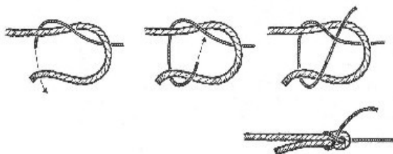
Schotstek
